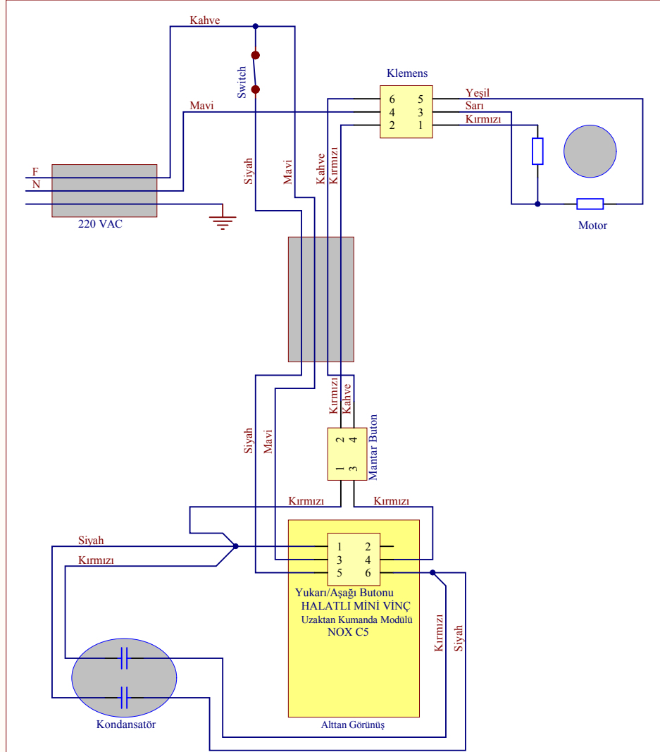
Uzaktan Kumanda Modülü Montaj Edilmiş Şekil
