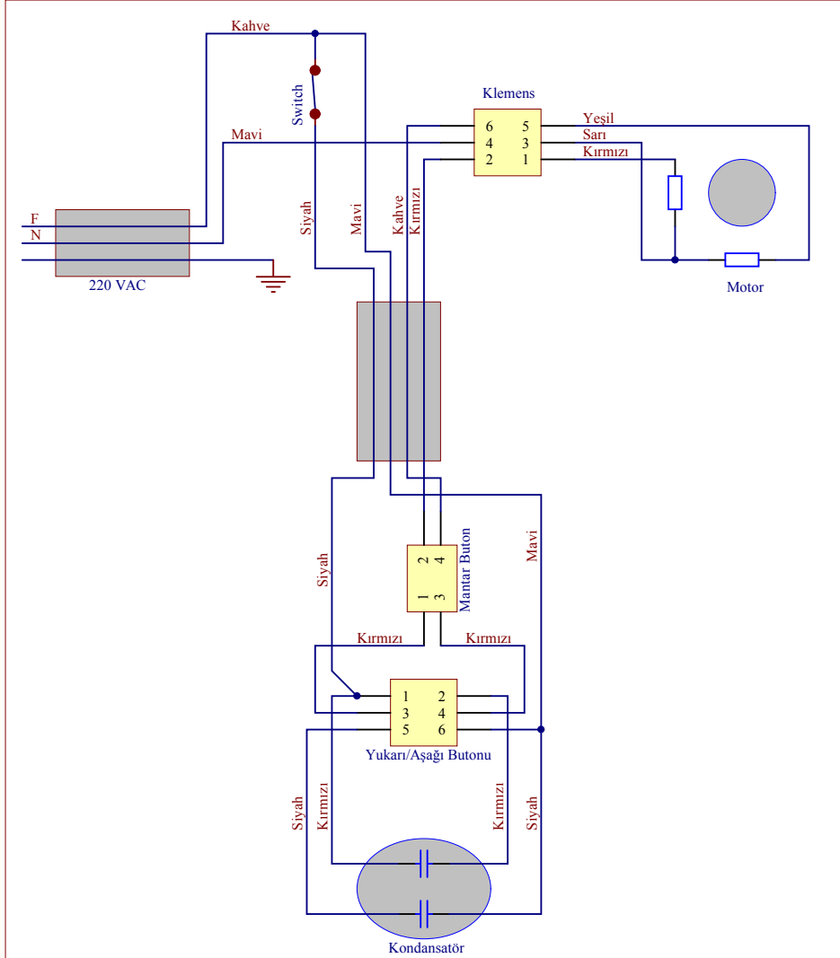
Vinç Orjinal Bağlantı Şekli
